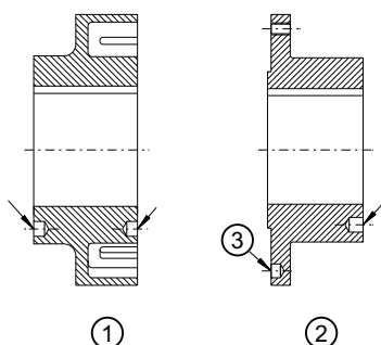
Image 5-4: Position du trou d'équilibrage pour l'équilibrage à deux plans
