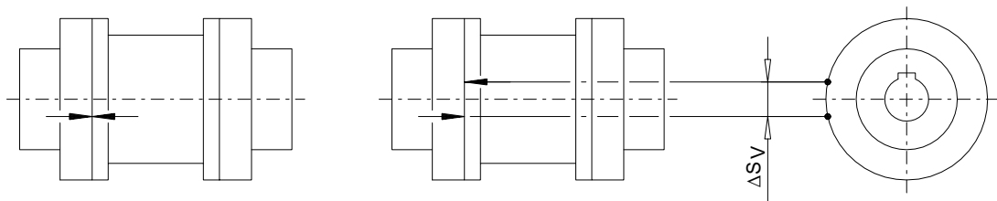
Image 8-1: Repères pour déterminer le jeu angulaire
