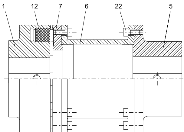
Image 3-1: Types H et HDS
