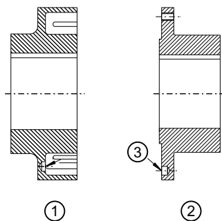
Image 5-3: Position du trou d'équilibrage pour l'équilibrage à un plan
