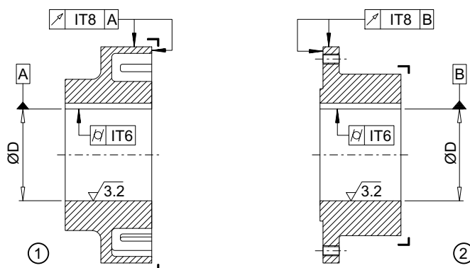
Image 5-1: Tolérances pour alésage de finition
