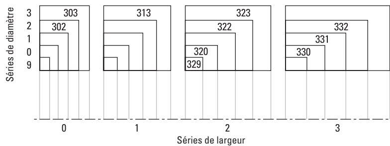
Fig. 31. Système ISO original de désignation.
