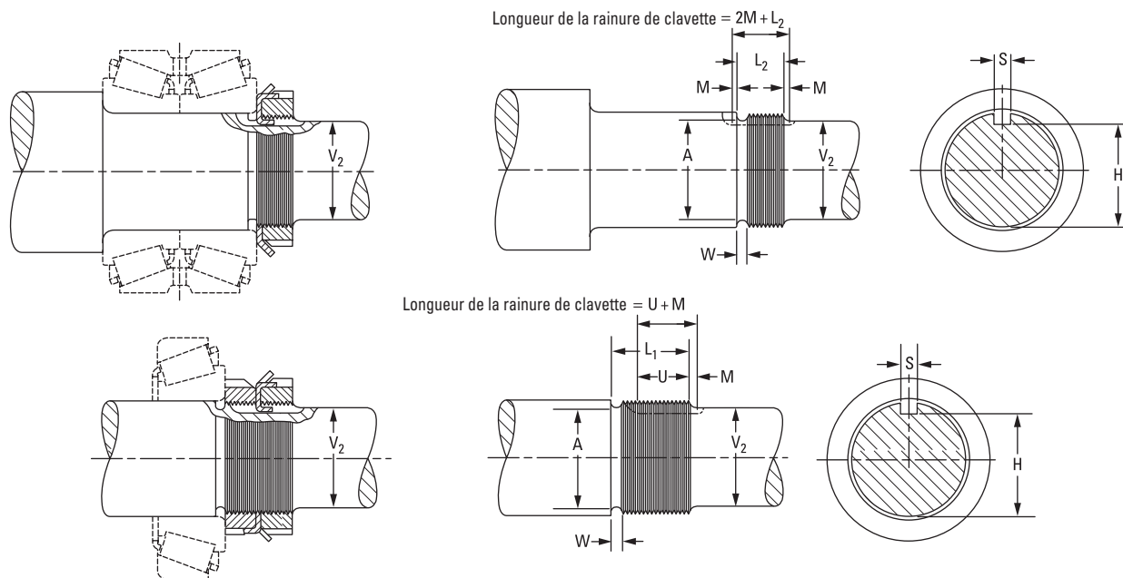
Fig. 55. Ecrus, rondelles-freins et rondelles à languette.
