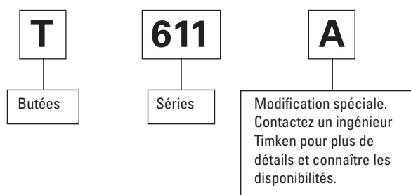
Fig. 41. Nomenclature des butées à rouleaux côniques.
