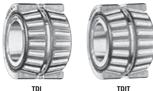
Fig. 4. Roulements à cône double à deux rangées.
