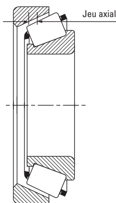
Fig. 14. Jeu interne – Jeu axial.
