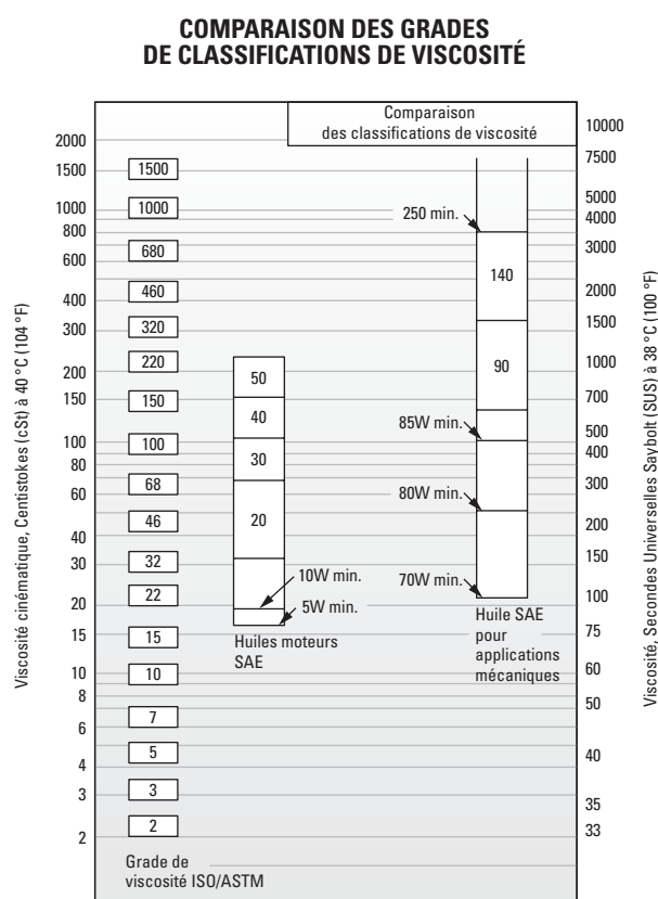
Fig. 21. Comparaison entre les grades ISO/ASTM (ISO 3448/ ASTM D2442) et les grades SAE (huiles SAE J 300-80 pour carters moteurs, huiles SAE J 306-81 pour ponts et transmission manuelle).
