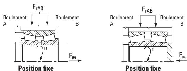
Conception (charge axiale extérieure, F_{ae} , sur roulement A)
