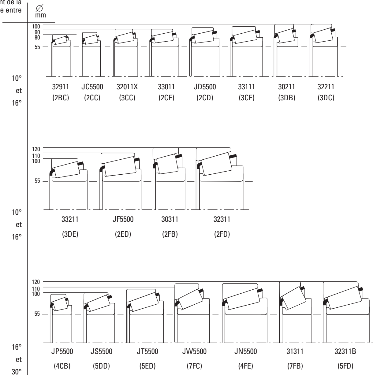
Fig. 29. Table de comparaison des sections d'un roulement de 55 mm (2,1654 po) de diamètre d'alésage.
