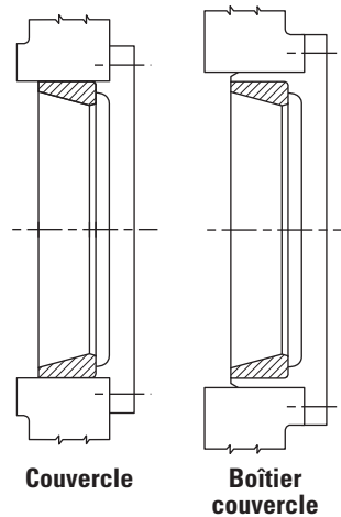
Fig. 10. Dispositifs de réglage de roulement – Montage direct.
