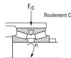
Roulement flottant
