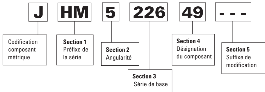
Fig. 27. Nomenclature du système de désignation des roulements J-Line.
