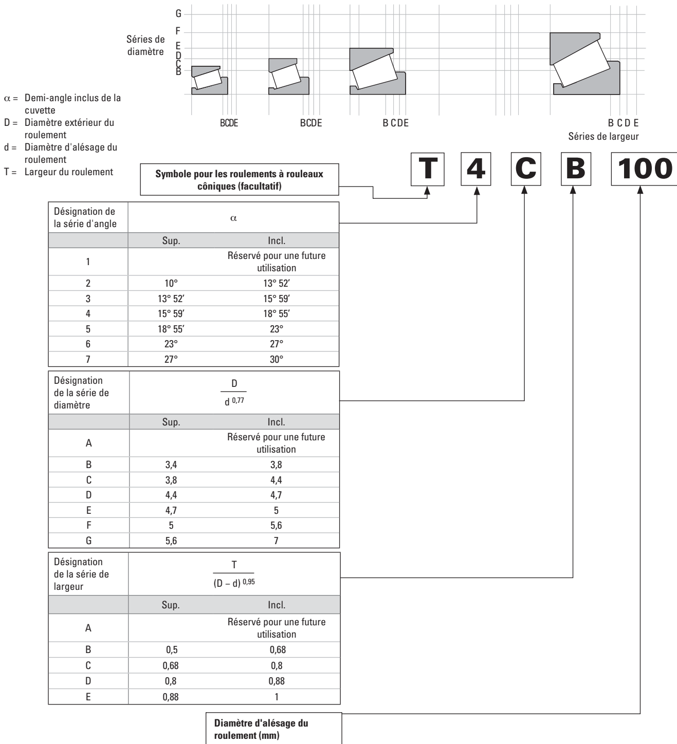
Fig. 32. Système de désignation ISO 355
