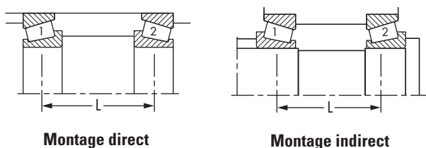
Fig. 16. Montage direct et indirect.
