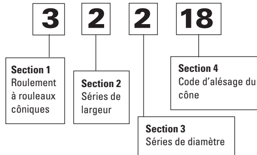
Fig. 30. Nomenclature du système ISO original de désignation des roulements.
