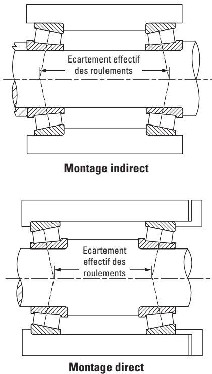
Fig. 9. Comparaison de la rigidité entre un montage direct et un montage indirect.
