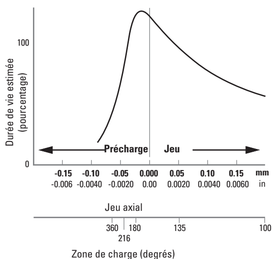
Fig. 13. Courbe classique de durée de vie vs réglage.
