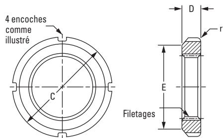
Fig. 49. Ecrous (filetages ISO 965/1, classe 5H).
