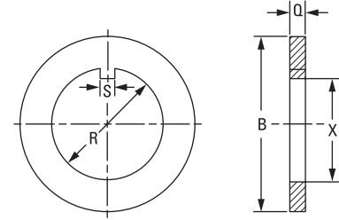
Fig. 54. Rondelles à languette.
