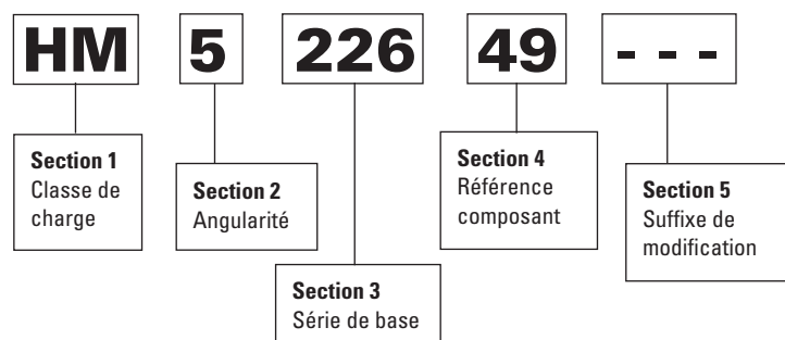
Fig. 26. Nomenclature du système de désignation ABMA des roulements en cotes pouces.
