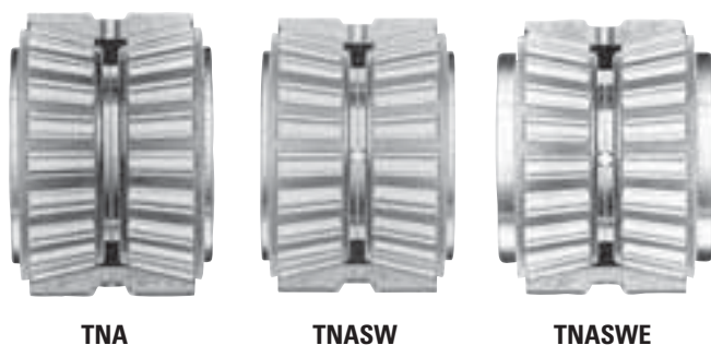
Fig. 5. Roulements non réglables à deux rangées.
