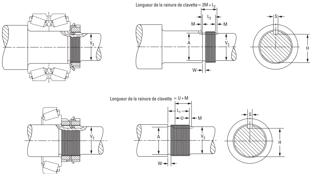
Fig. 56. Ecrus, rondelles freins et rondelles à languette.
