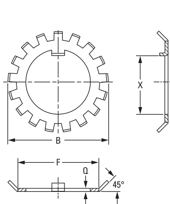
Fig. 53. Rondelles-freins.
