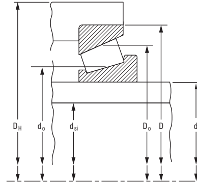
Fig. 15. Paramètres dimensionnels ayant une incidence sur l'ajustement et les effets de température .
