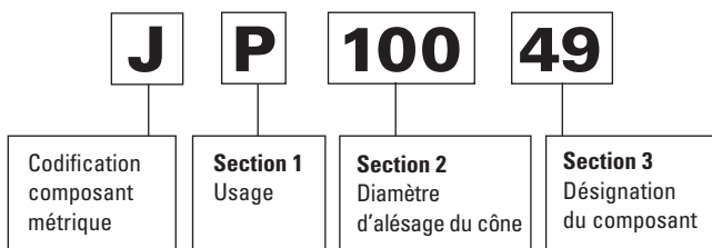
Fig. 28. Nomenclature du système de désignation des roulements avec préfixe J.
