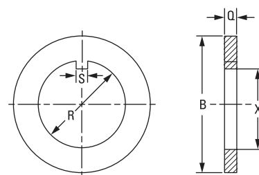
Fig. 51. Rondelles à languette.
