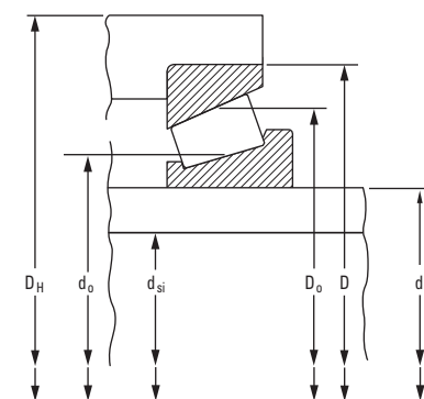
Fig. 12. Paramètres de calcul de l'effet de l'ajustement sur le réglage.
