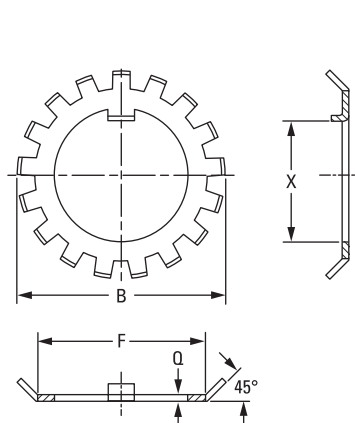
Fig. 50. Rondelles-freins.
