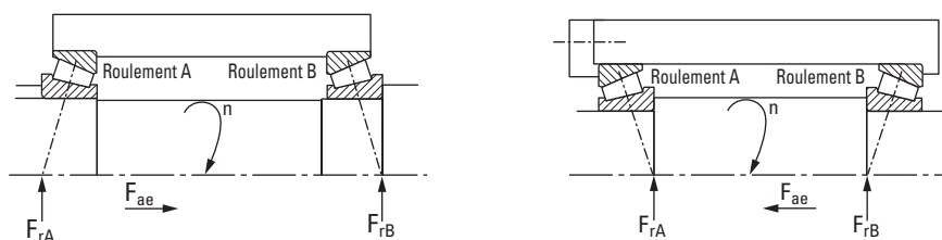
Conception (charge axiale extérieure, F_{ae} , sur le roulement A)
