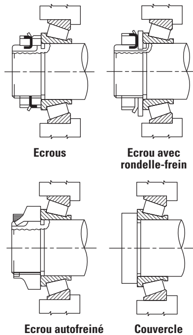
Fig. 11. Dispositifs de réglage de roulement – Montage indirect.
