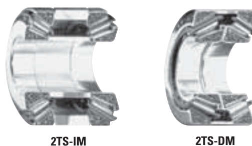
Fig. 7. Assemblages entretoisés.
