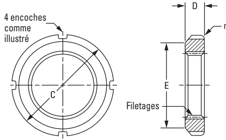
Fig. 52. Ecrus (filetages ISO 965/1, classe 5H).
