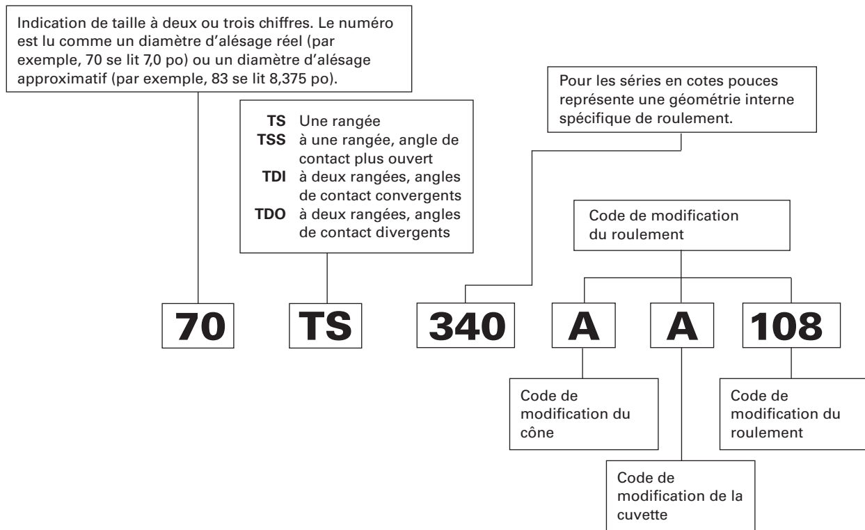
Fig. 33. Nomenclature historique des roulements à rouleaux côniques.
