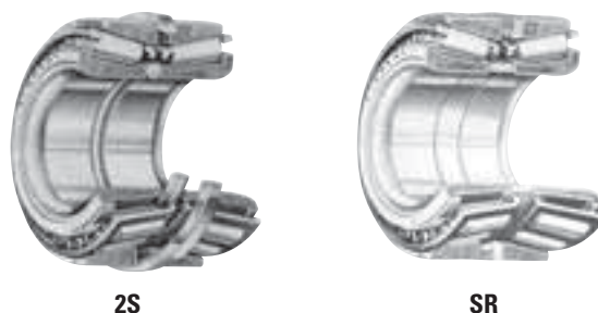
Fig. 6. Assemblages entretoisés.
