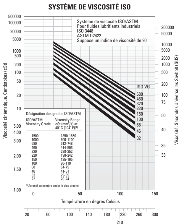
Fig. 22. Système de grades de viscosité des huiles industrielles.
