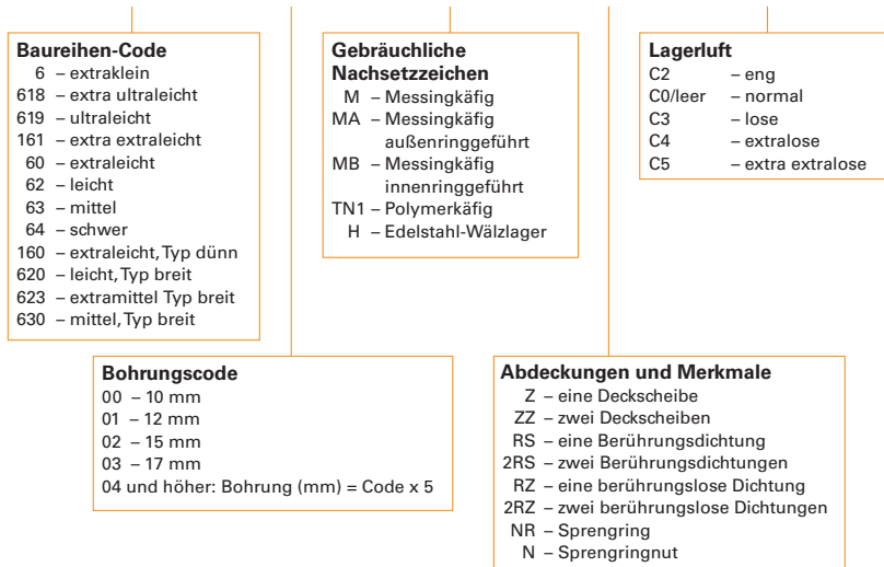
Abb. 1. Bezeichnungssystem für Rillenkugellager
