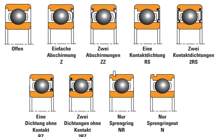
Abb. 4. Rillenkugellager-Varianten
